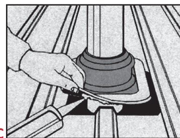
C. APPLIQUER LE MASTIC (FOURNI DANS LE KIT) SOUS L'EMBASE DU MANCHON. C. BRENG AAN ONDERZIJDE BEVESTIGINGSRAND EEN NEUTRALE SILICONENKIT AAN
