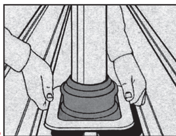
B. ENGAGER LE MANCHON SUR LE CONDUIT ET LE FAIRE GLISSER JUSQU'AU PROFIL. B. SCHUIF DOORVOER OVER DE PIJP
