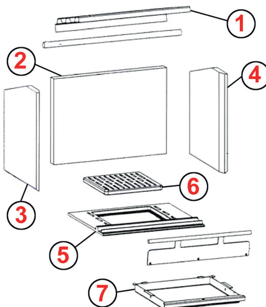
2 PLAQUE ARRIÈRE ACHTERPLAAT | DIP 0052116
