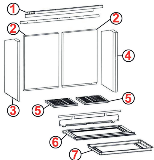
7 CENDRIER ASBAK DIP 0019785
