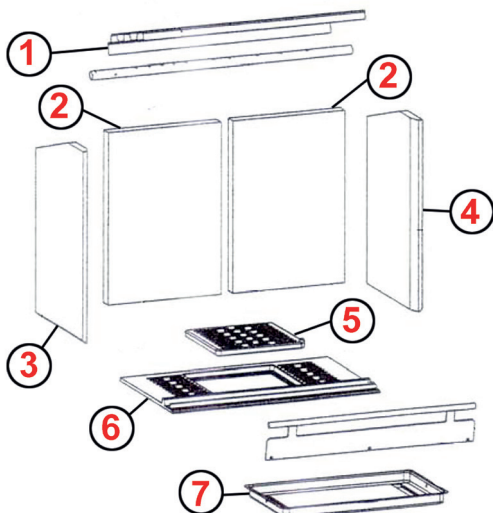
7 CENDRIER ASBAK DIP 0047572
