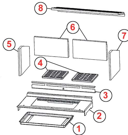
6 BRIQUE FOND ACHTER STEEN DIP 0052505
