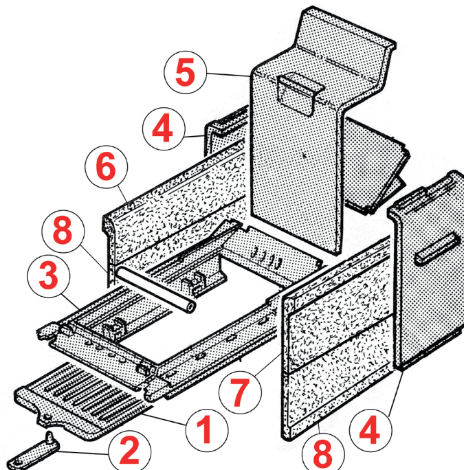
6 47166 DIP 0047166 BRIQUE GAUCHE HAUTE STEEN LINKS BOVEN
