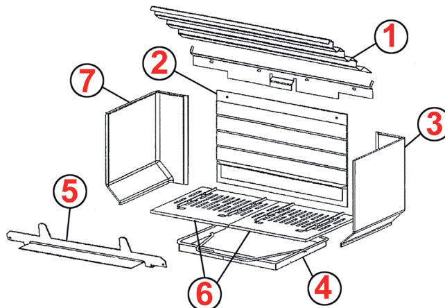
6 GRILLE ROOSTER DIP 0018632 2PCS - 2STK
